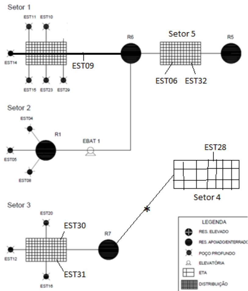
Figura 18 – Fluxograma do SAA.
