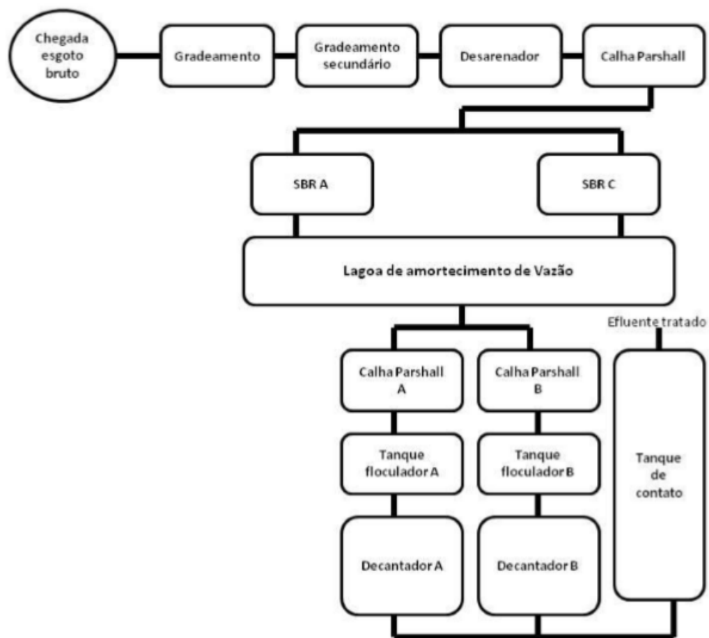
Figura 28 – Unidades de Tratamento da ETE Alvorada-Viamão.
