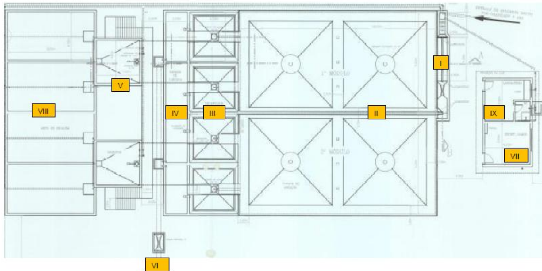
Figura 23 – Unidades de Tratamento da ETE Buena Vista.
