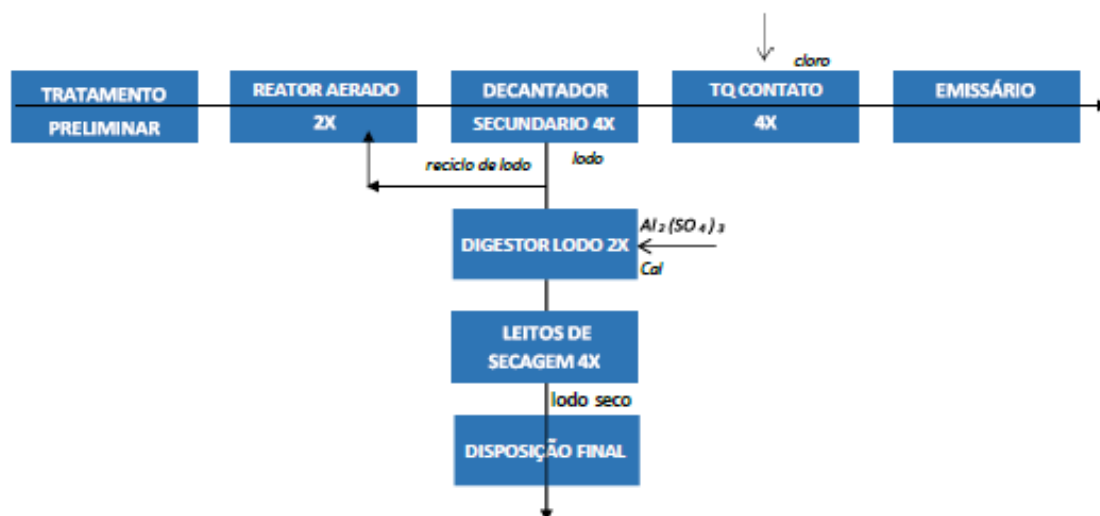
Figura 26 – Fluxograma da ETE componente do SES Buena Vista.
