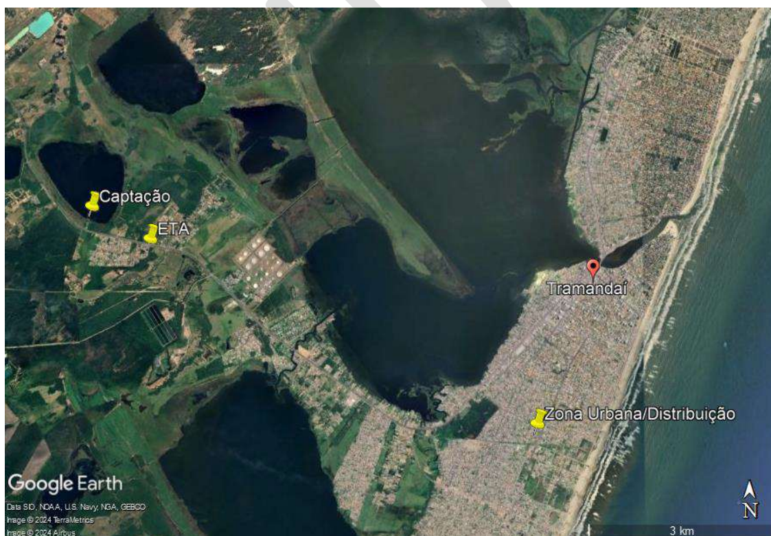
Figura 22 – Pontos vulneráveis do SAA.
