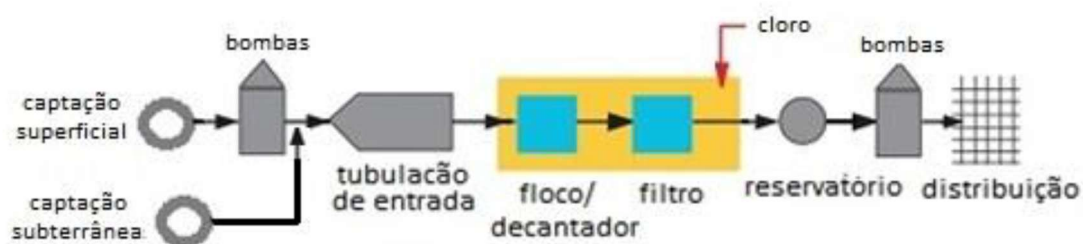
Figura 21 – Fluxograma do SAA.
