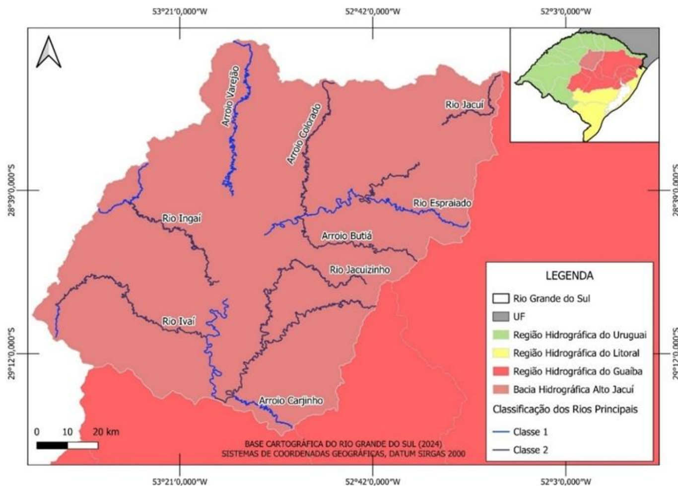
Figura 8 – Enquadramento dos rios principais na Bacia Hidrográfica Alto Jacuí.
