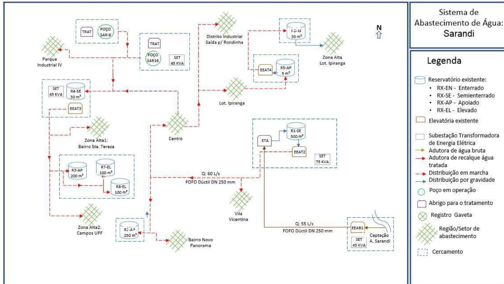
Figura 18 – Fluxograma do SAA.
