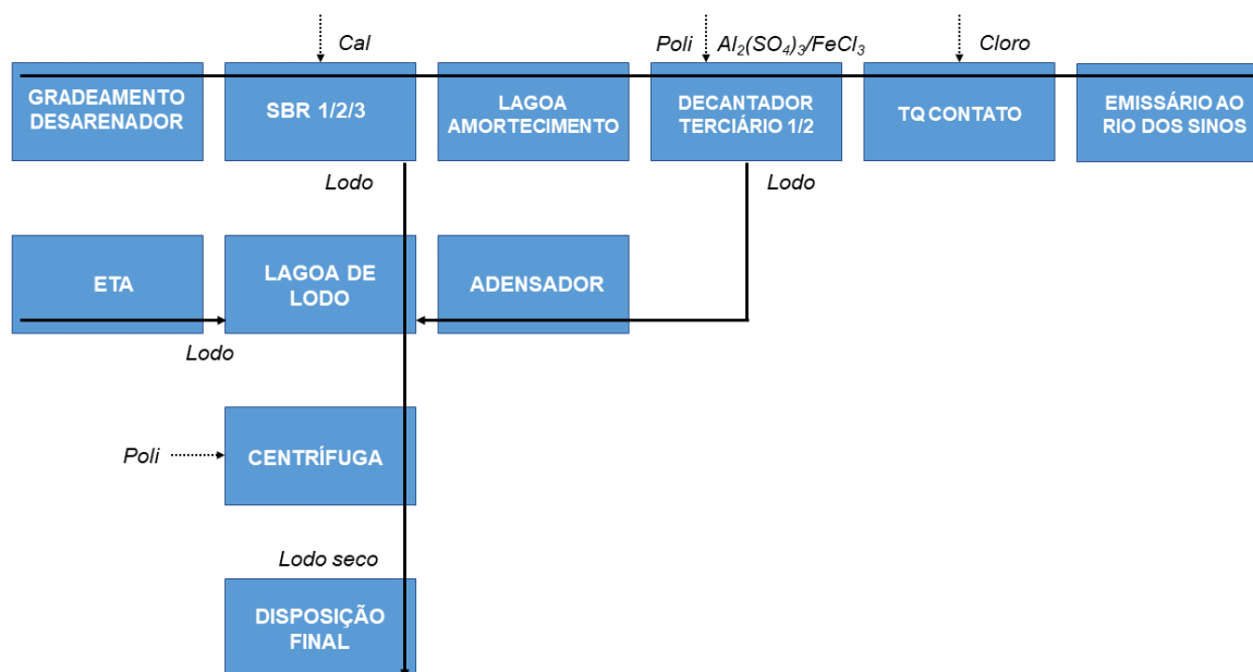
Figura 28 – Fluxograma da ETE componente do SES Esteio-Sapucaia do Sul.
