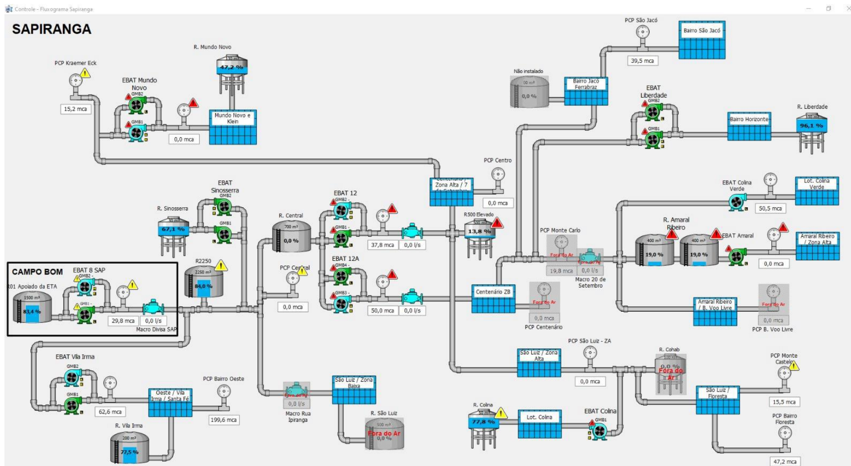
Figura 19 – Fluxograma do SAA.
