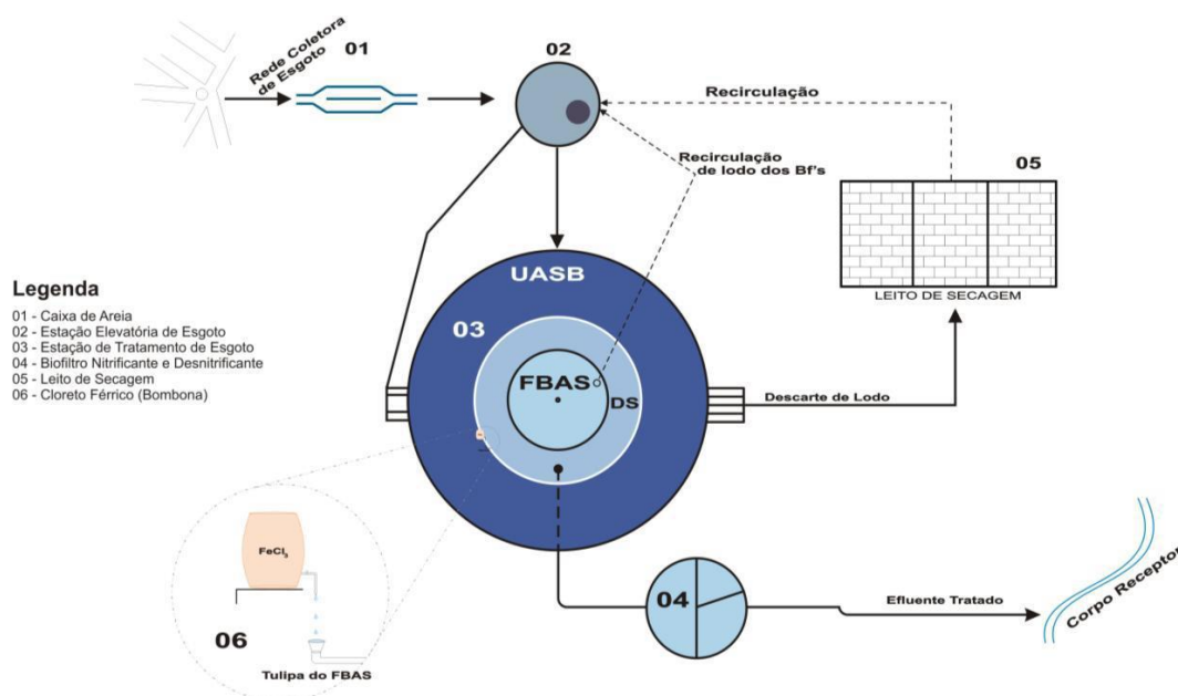
Figura 20 – Fluxograma ETE Passo da Cruz.
