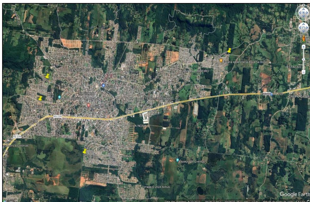
Figura 18 – Áreas urbanas não atendidas pelo SAA.
