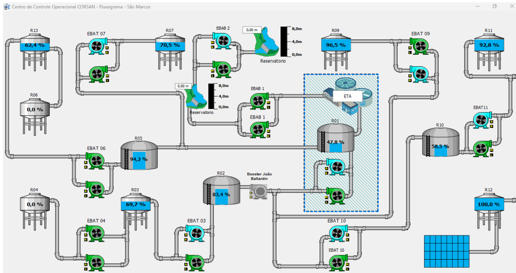
Figura 18 – Fluxograma do SAA.
