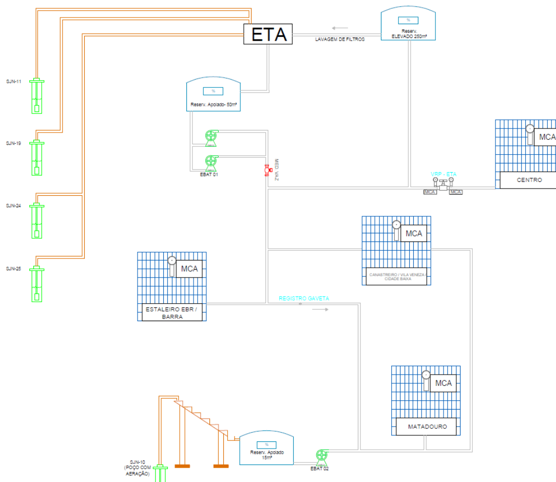
Figura 23 – Fluxograma do SAA.
