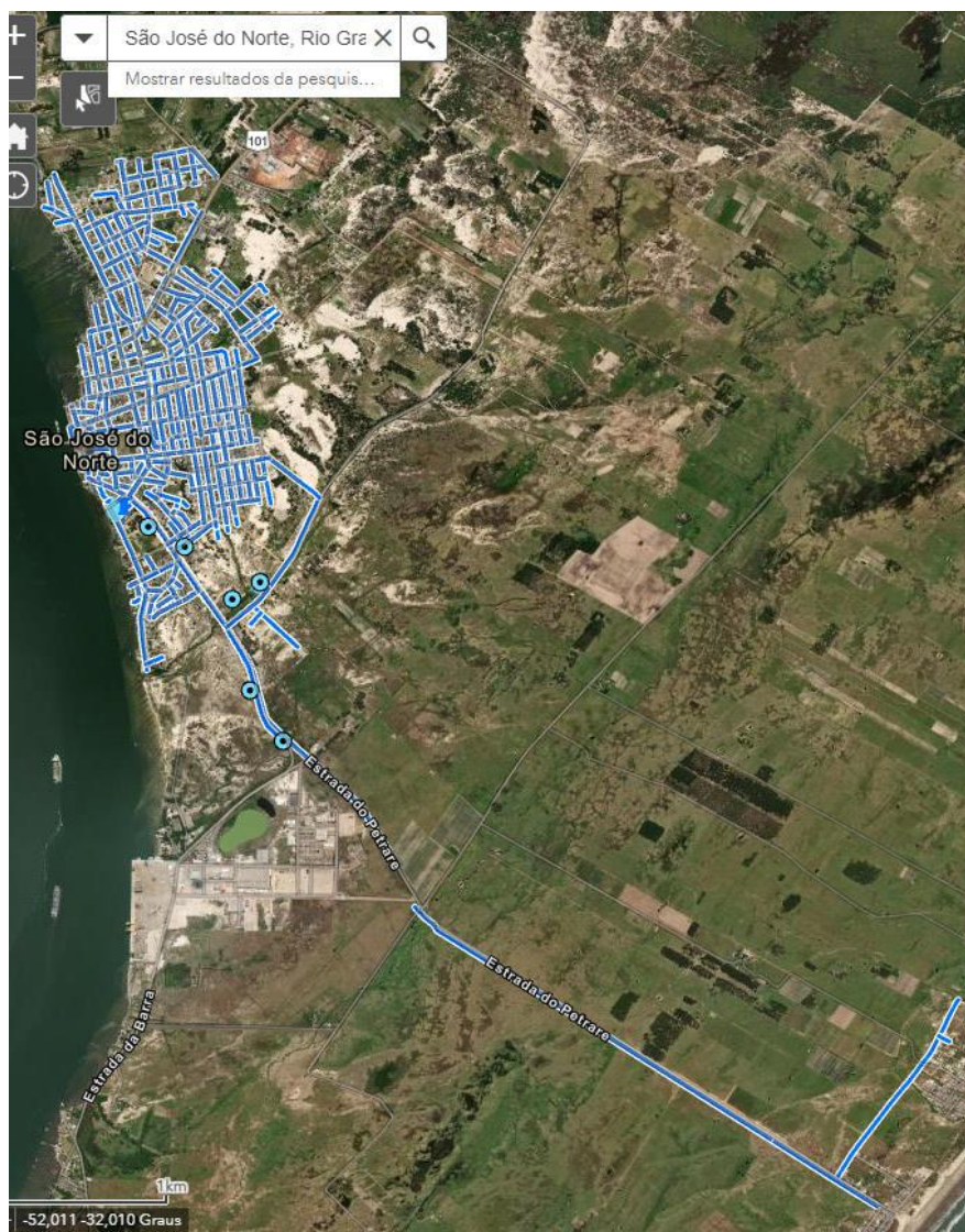
Figura 21 – Mapa adutoras e redes de distribuição de água (1).
