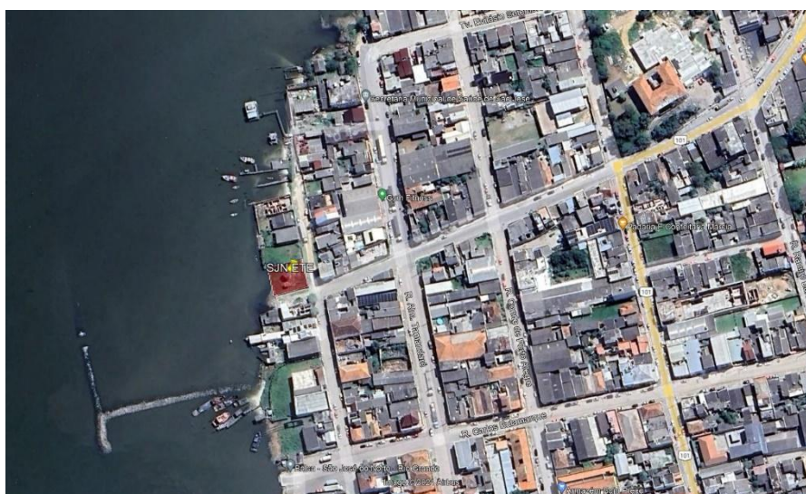
Figura 29 – Vista aérea da ETE São José do Norte.
