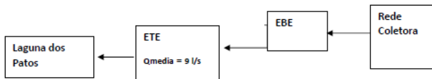
Figura 31 – Fluxograma da ETE e do SES.
