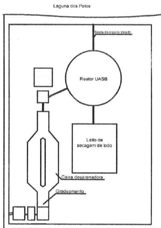
Figura 28 – Diagrama esquemático da ETE São José do Norte.
