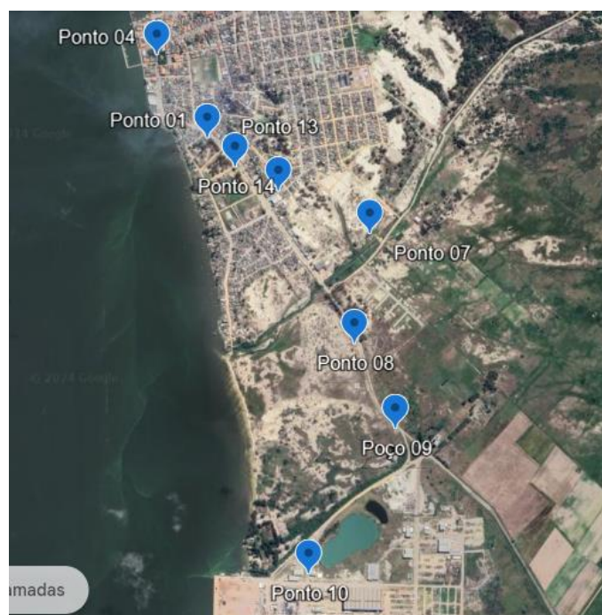
Figura 25 – Pontos vulneráveis SAA (2).
