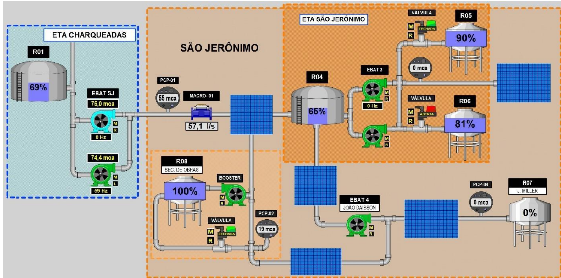
Figura 18 – Fluxograma do SAA.
