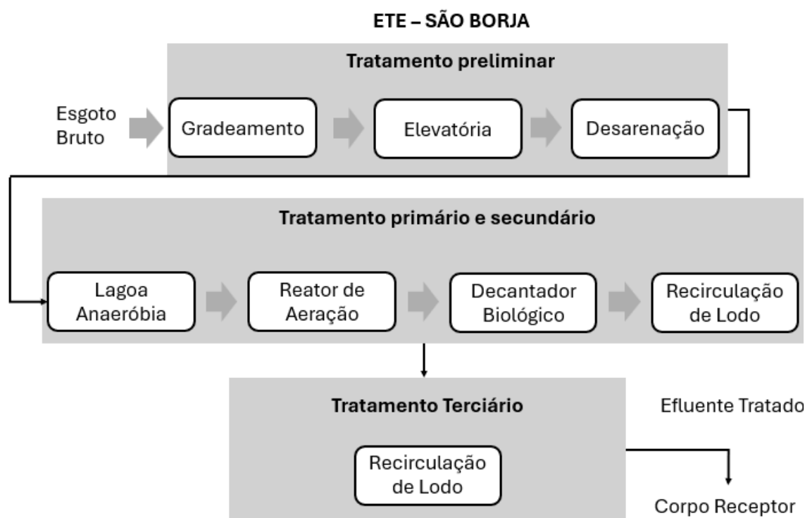
Figura 25 – Fluxograma do tratamento da ETE São Borja.
