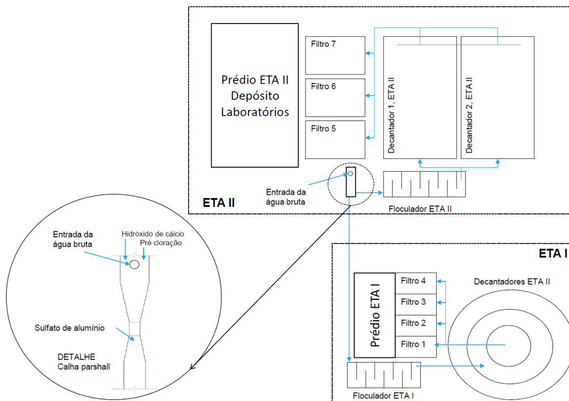
Figura 19 – Fluxograma do tratamento de água nas ETAS I e II de São Borja.
