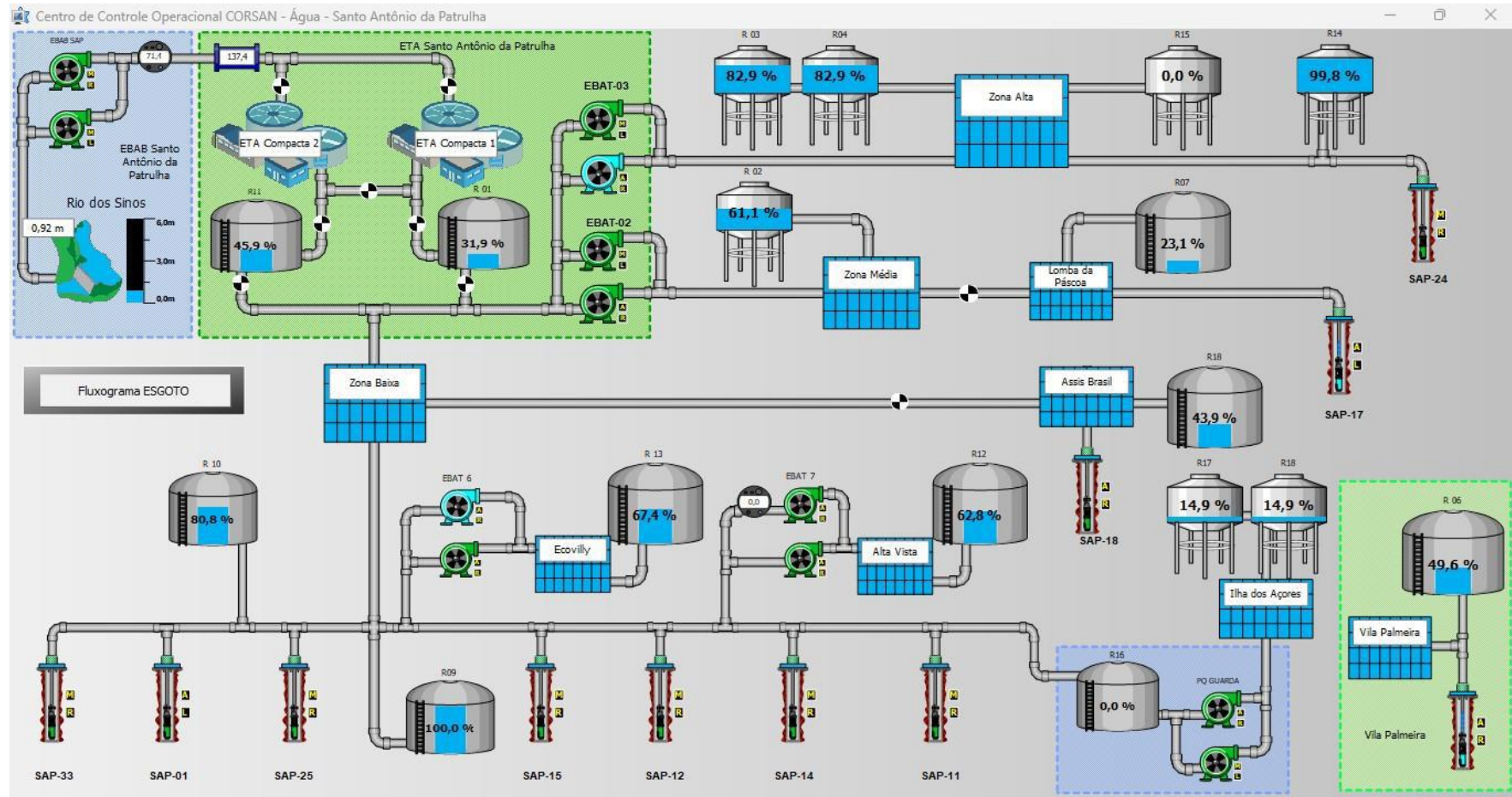
Figura 33 – Fluxograma do SAA.
