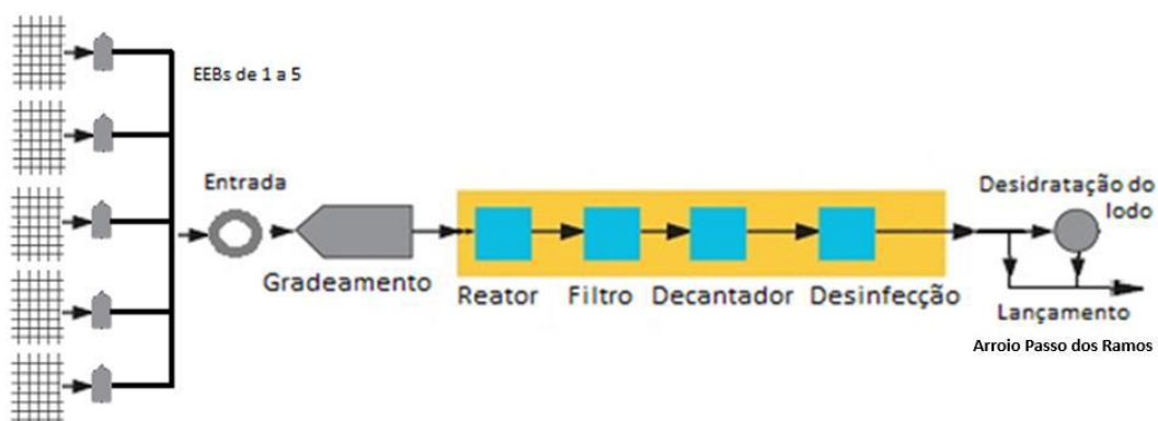
Figura 38 – Fluxograma do SES.
