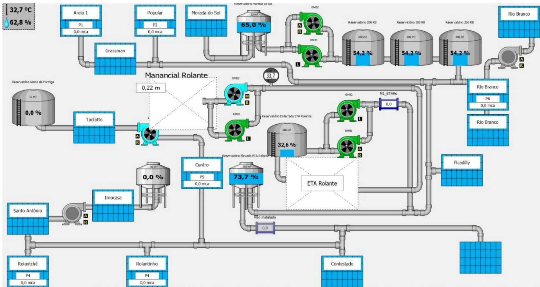
Figura 18 – Fluxograma do SAA.
