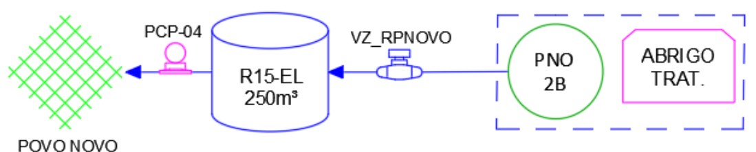
Figura 18 – Fluxograma operacional – Povo Novo.
