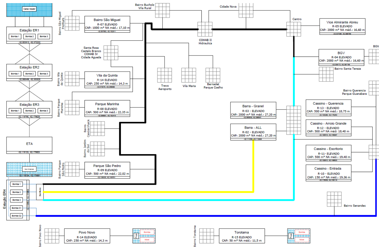
Figura 22 – Fluxograma do SAA.
