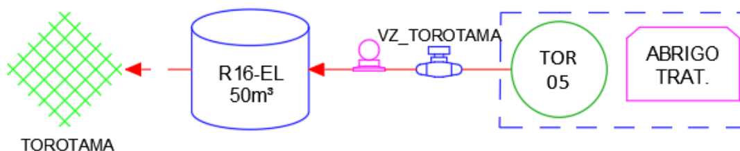
Figura 19 – Fluxograma operacional – Poço Torotama.
