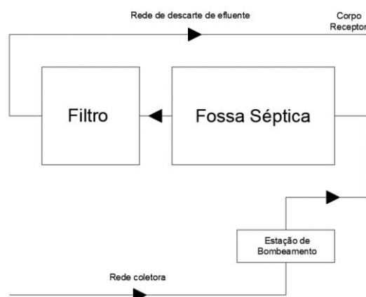
Figura 35 – Fluxograma esquemático do sistema Figueiras Parks.
