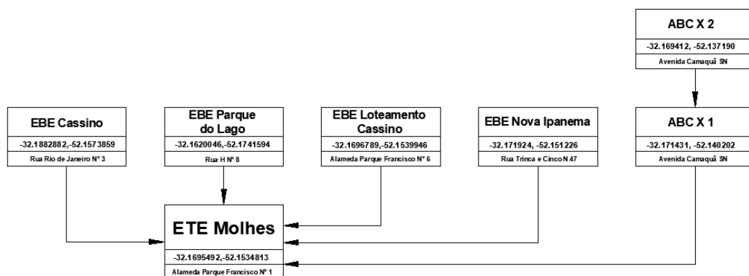
Figura 33 – Fluxograma esquemático do sistema Molhes.
