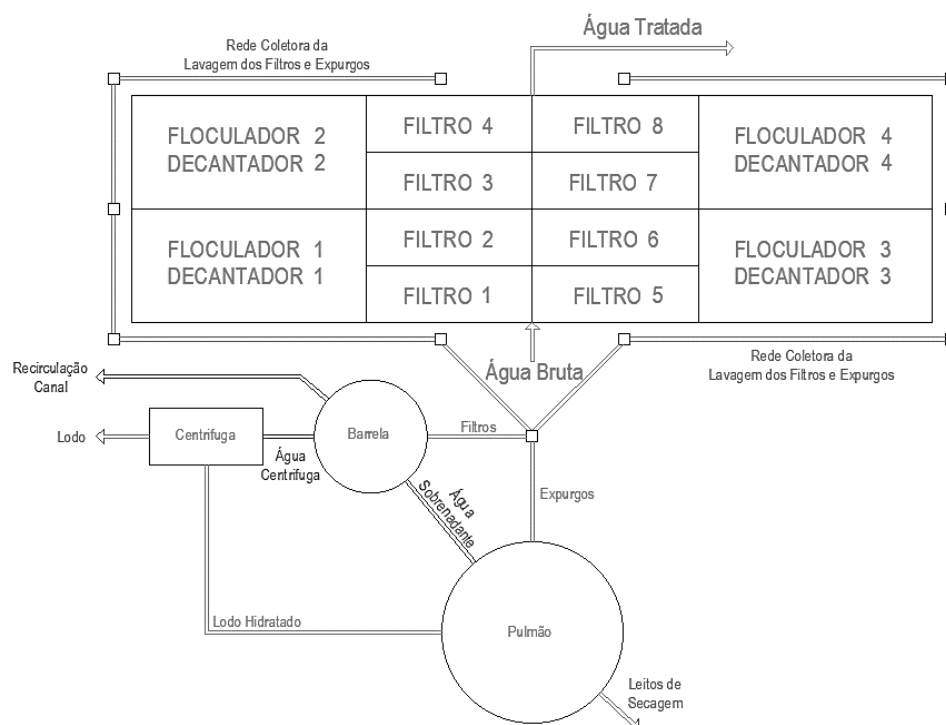
Figura 20 – Fluxograma esquemático operacional da ETA Rio Grande
