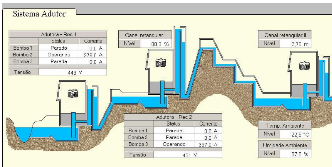
Figura 21 – Imagem extraída do software de operação do CCO Rio Grande, esquemático operacional de adução de água bruta de Rio Grande.
