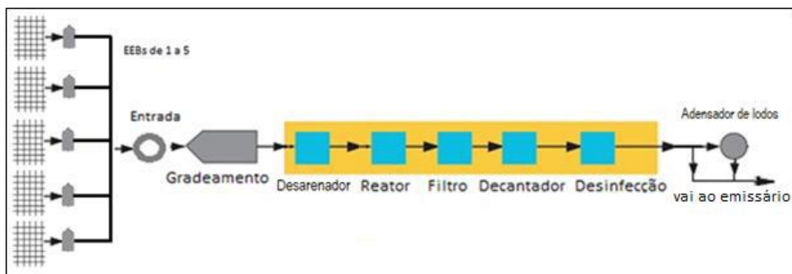
Figura 26 – Fluxograma da ETE e do SES.
