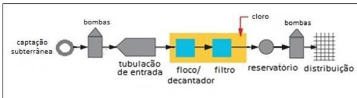
Figura 22 – Fluxograma do SAA.
