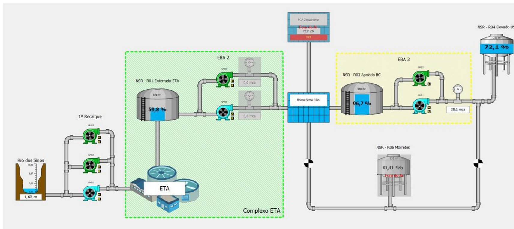
Figura 18 – Fluxograma do SAA.
