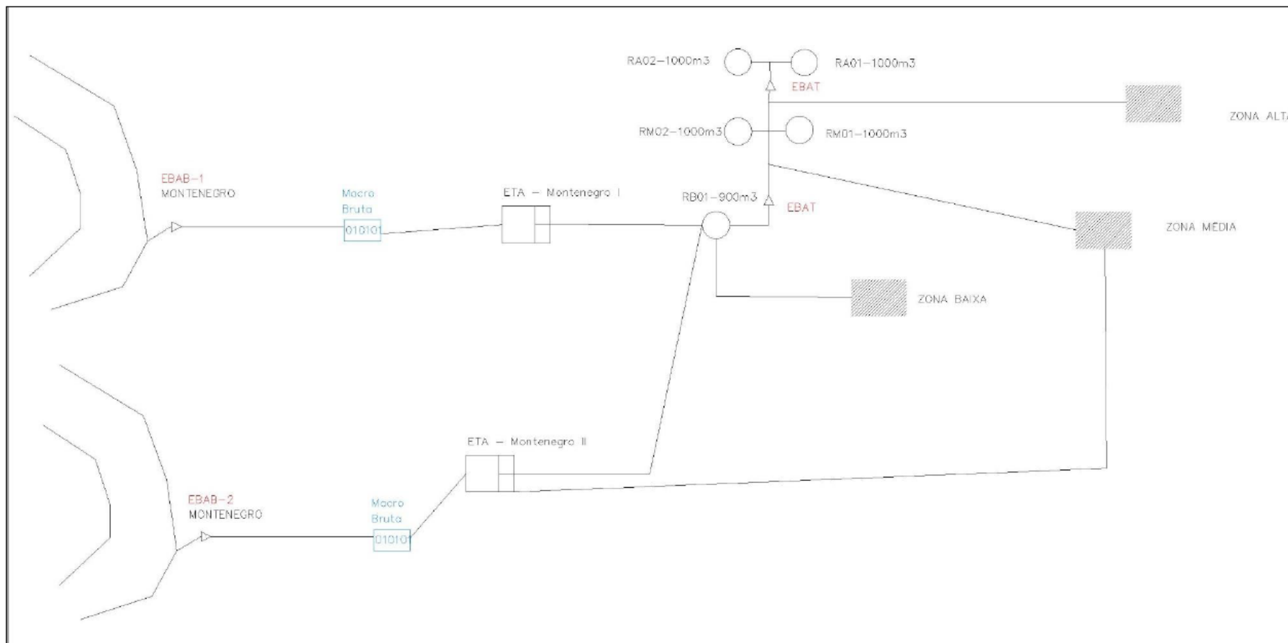
Figura 18 – Fluxograma do SAA (1).
