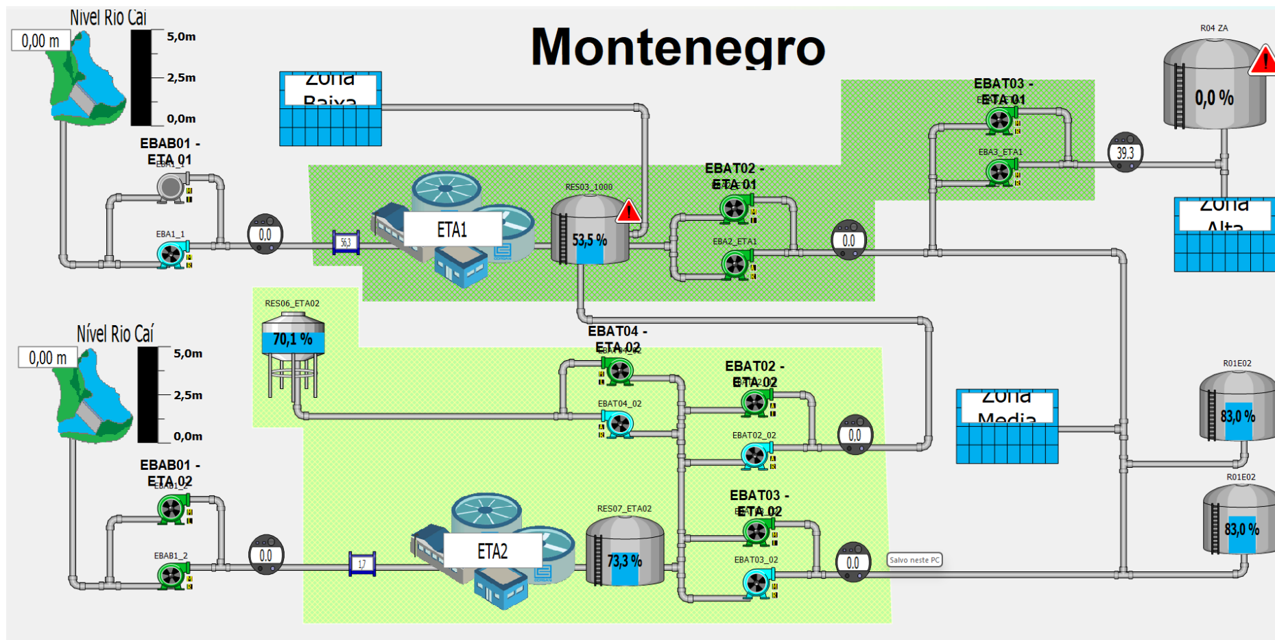
Figura 19 – Fluxograma do SAA (2).
