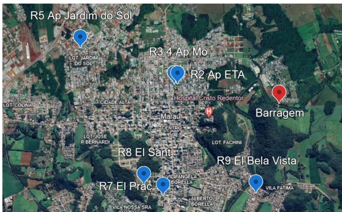
Figura 18 – Croqui do SAA de Marau – Reservação.
