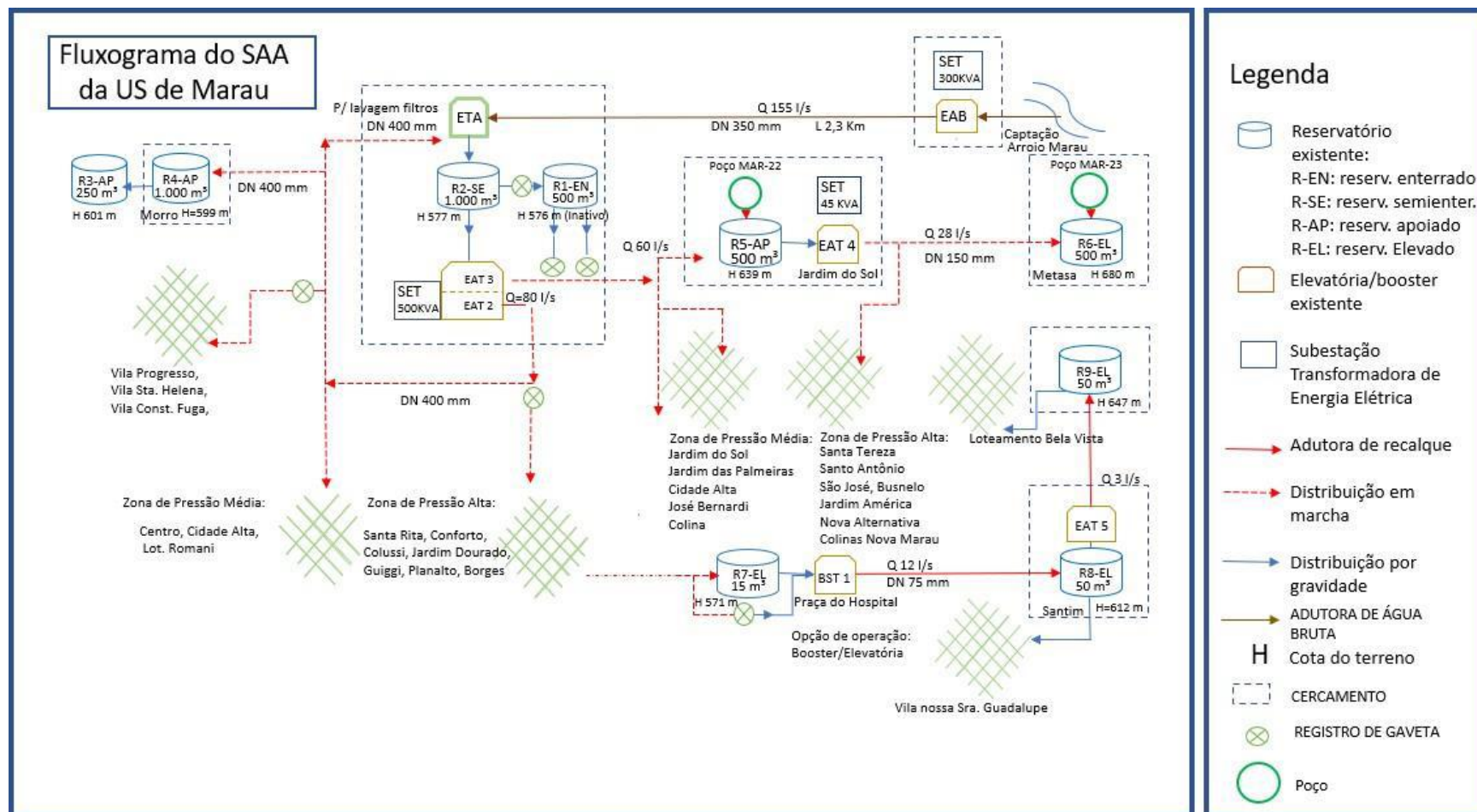
Figura 20 – Fluxograma do SAA.
