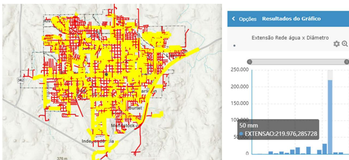
Figura 20 – Extensão de Rede de Água vs. Diâmetro.
