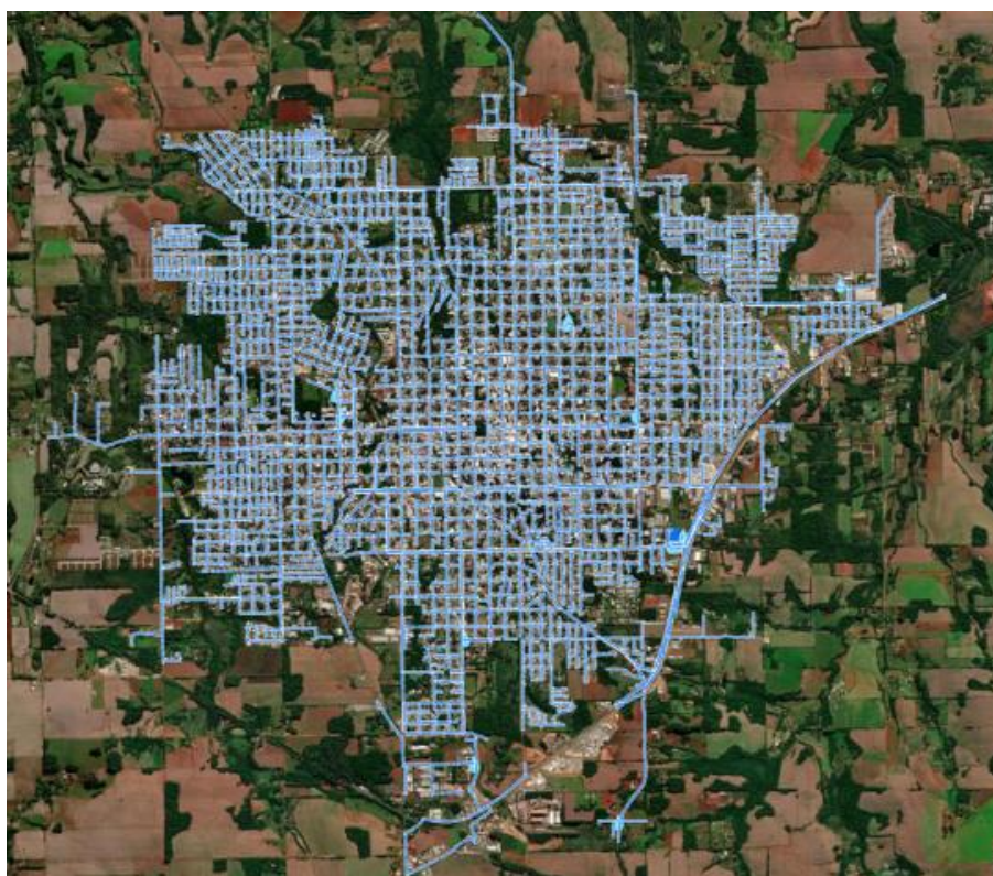
Figura 19 – Rede de Abastecimento de Ijuí.
