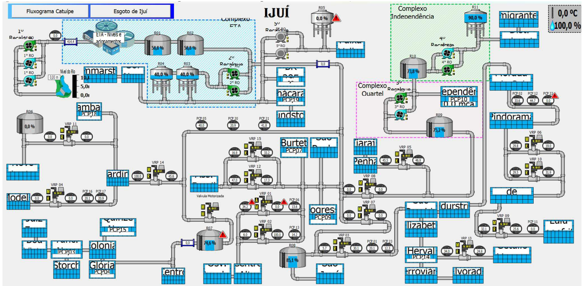
Figura 22 – Fluxograma do SAA.
