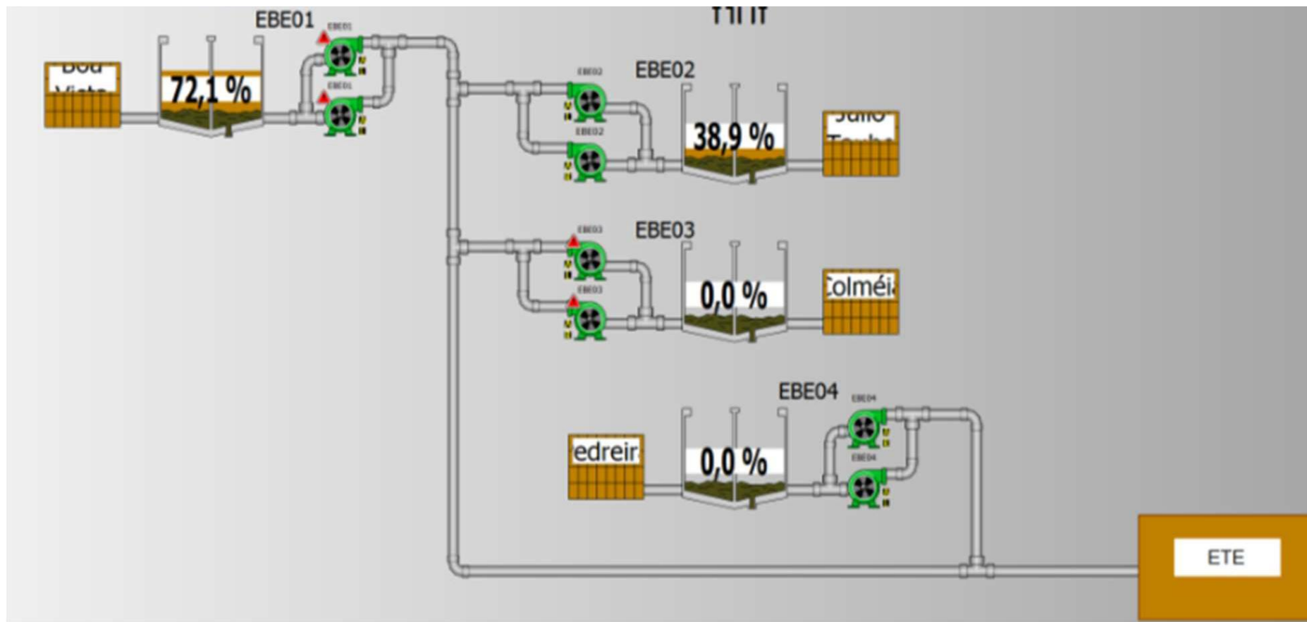
Figura 26 – Fluxograma do SES.
