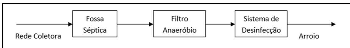
Figura 20 – Fluxograma ETE.
