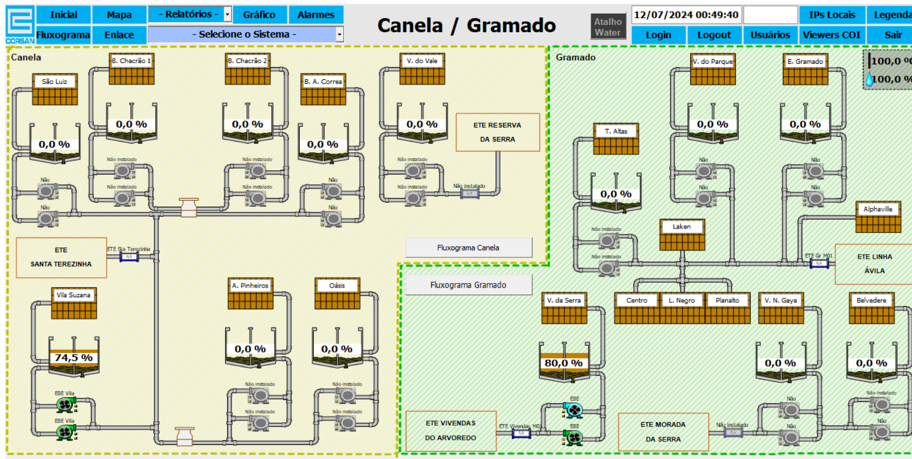
Figura 21 – Fluxograma da ETE e do SES.
