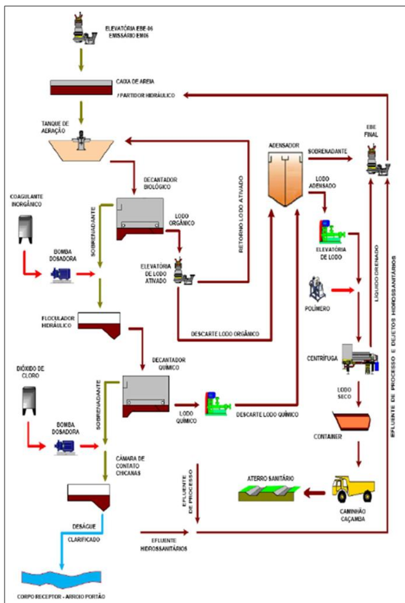
Figura 21 – Fluxograma da ETE Estância Velha.
