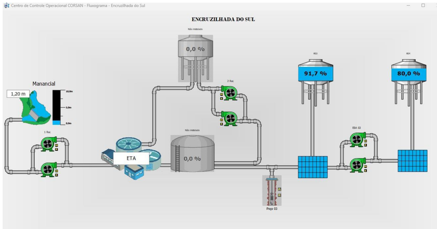
Figura 19 – Fluxograma do SAA.
