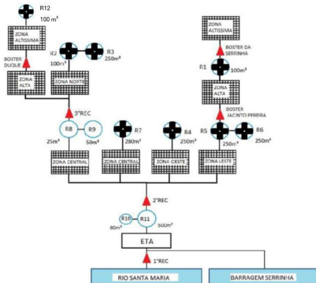
Figura 20 – Croqui da distribuição de água no município de Dom Pedrito.
