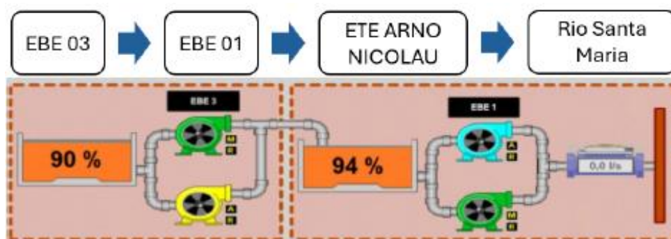
Figura 26 – Fluxograma simplificado do SES Dom Pedrito.
