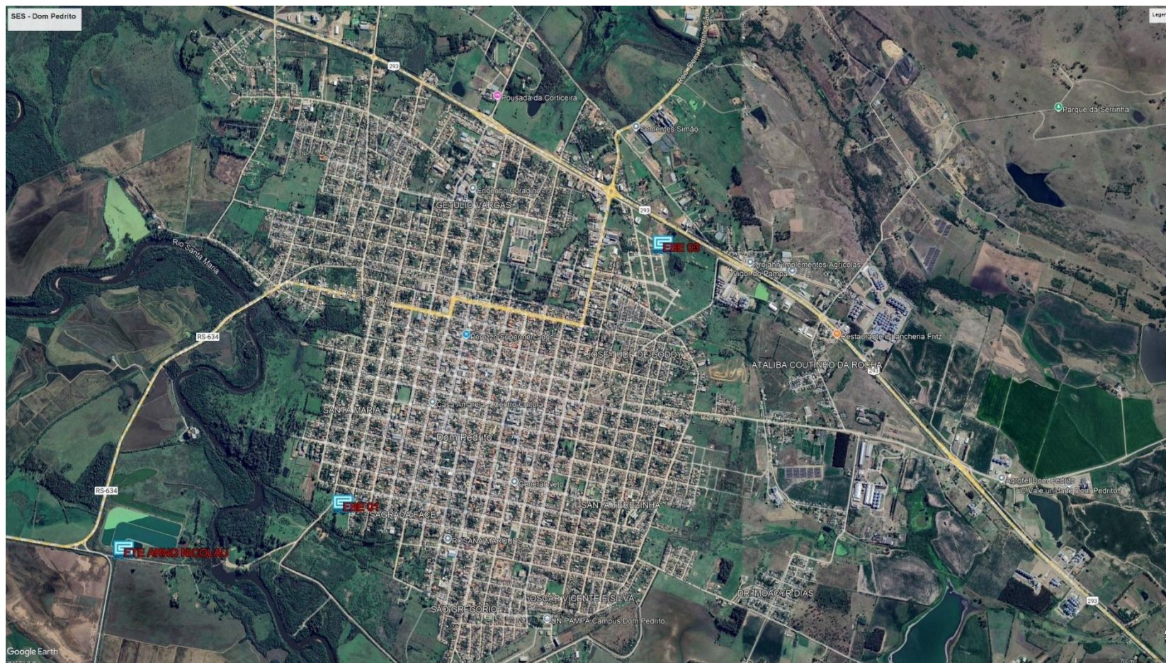
Figura 24 – Localização das EBEs e ETE do SES Dom Pedrito. Em operação: EBE 01 e EBE 03.
