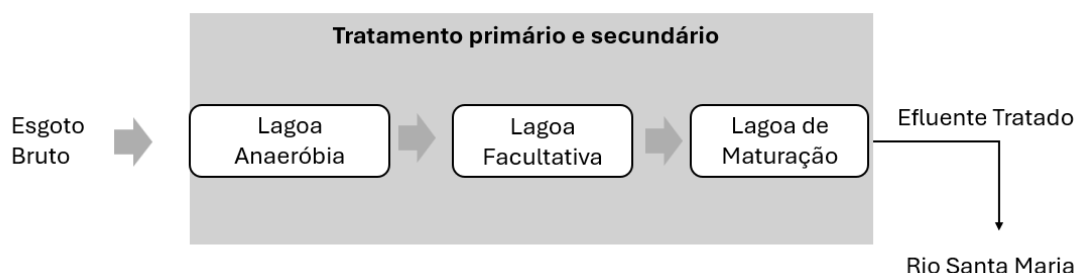
Figura 25 – Fluxograma simplificado do tratamento na ETE Arno Nicolau Heck.
