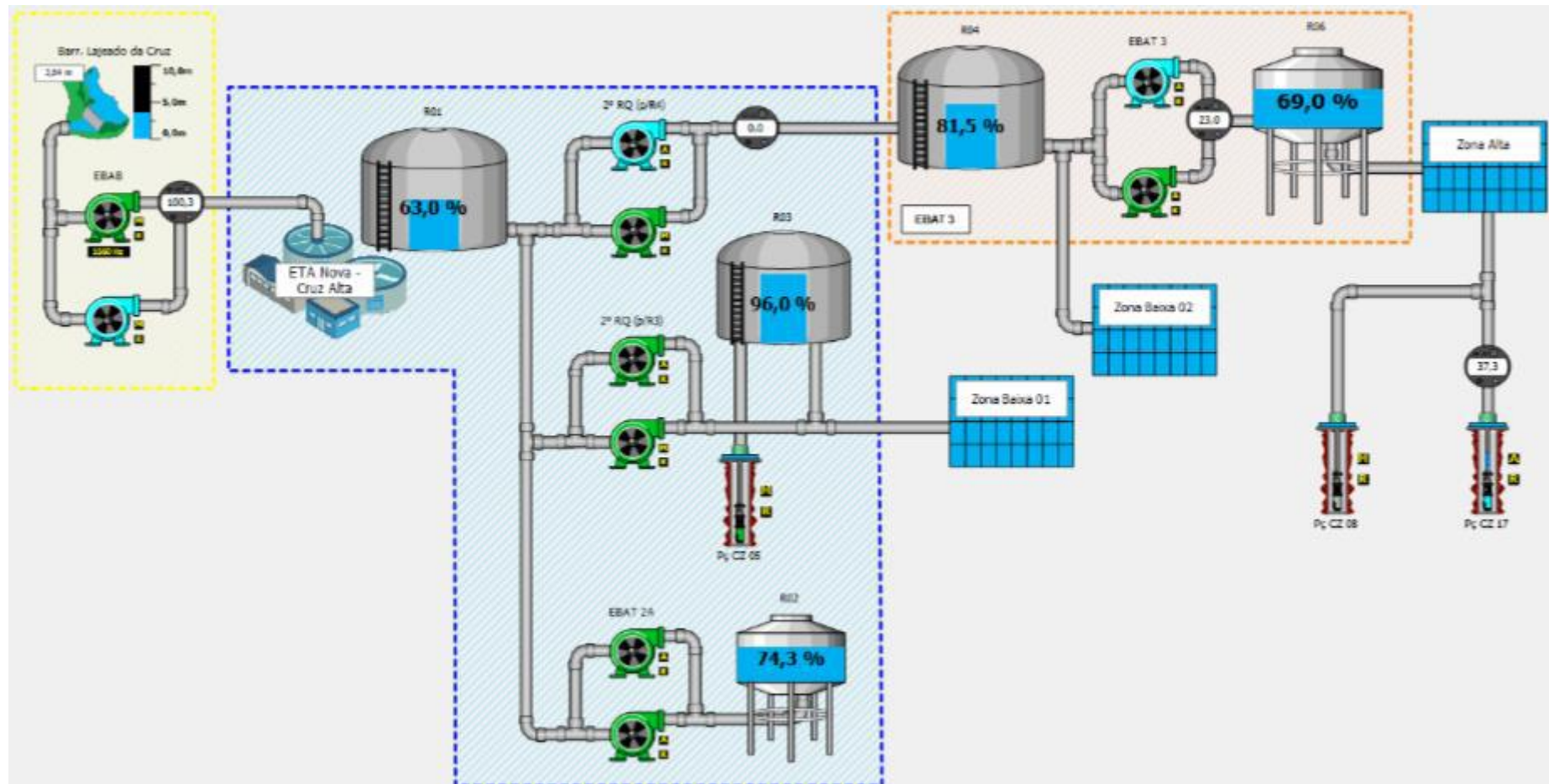
Figura 20 – Fluxograma do SAA.
