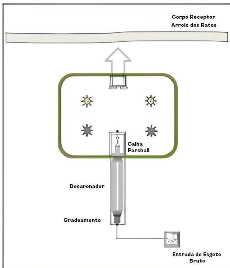
Figura 24 – Fluxograma da ETE.
