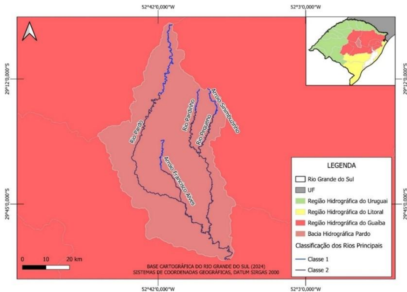
Figura 8 – Enquadramento dos rios principais na Bacia Hidrográfica Pardo.
