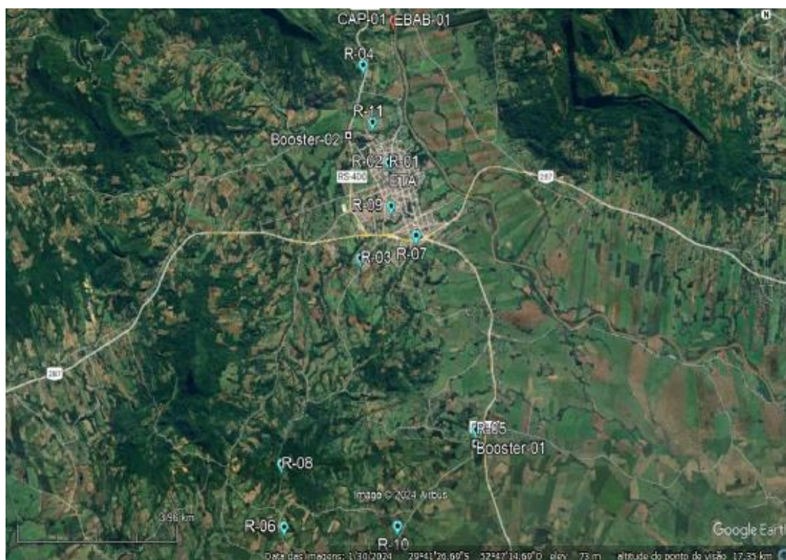
Figura 20 – Pontos vulneráveis do SAA.
