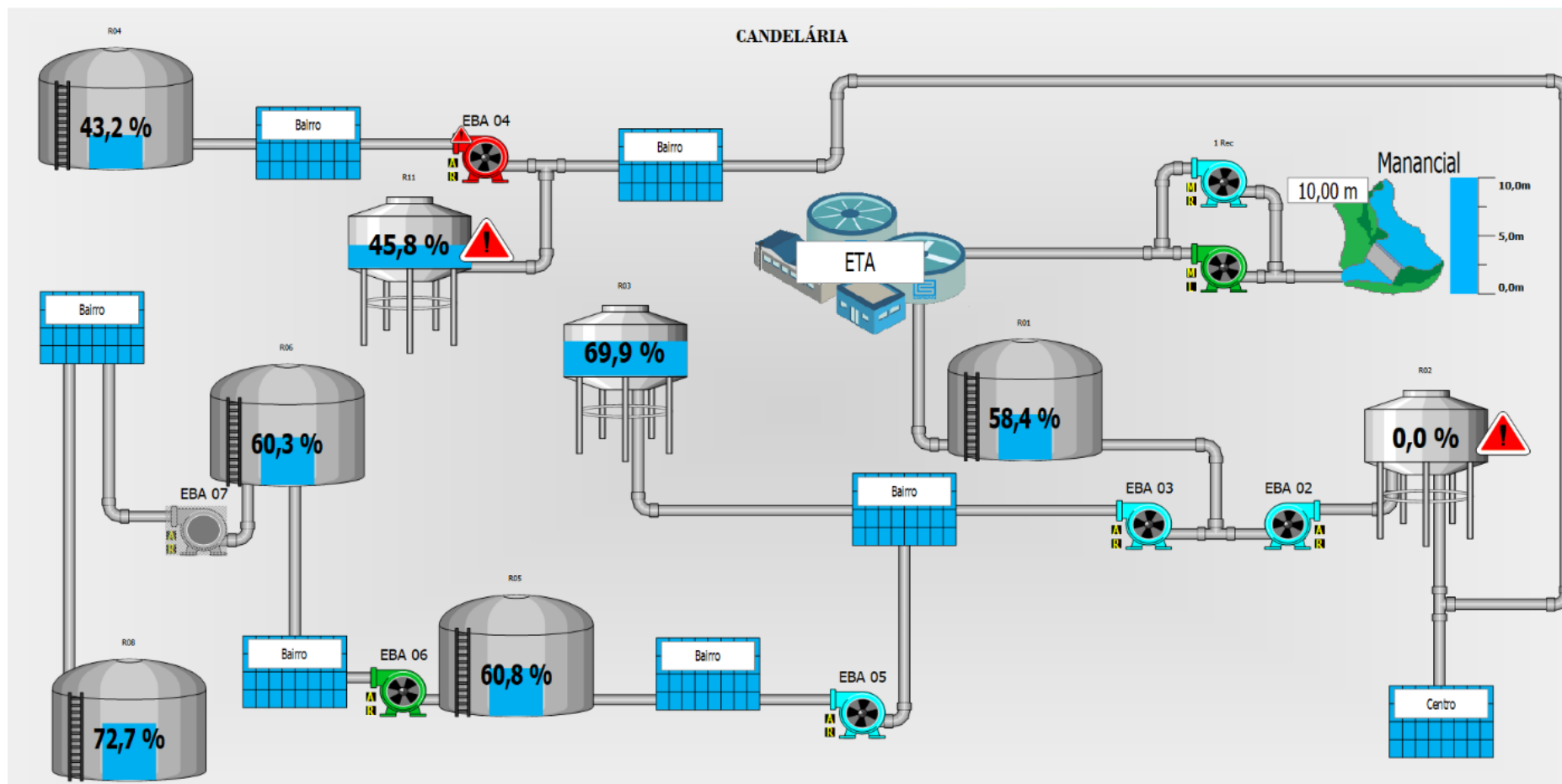
Figura 18 – Fluxograma do SAA – COI.
