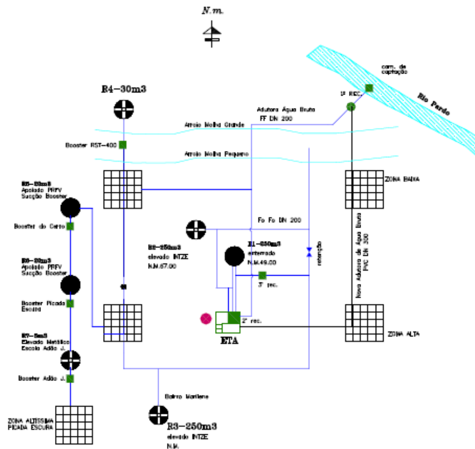
Figura 19 – Fluxograma do SAA.
