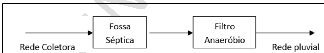
Figura 19 – Fluxograma ETE.
