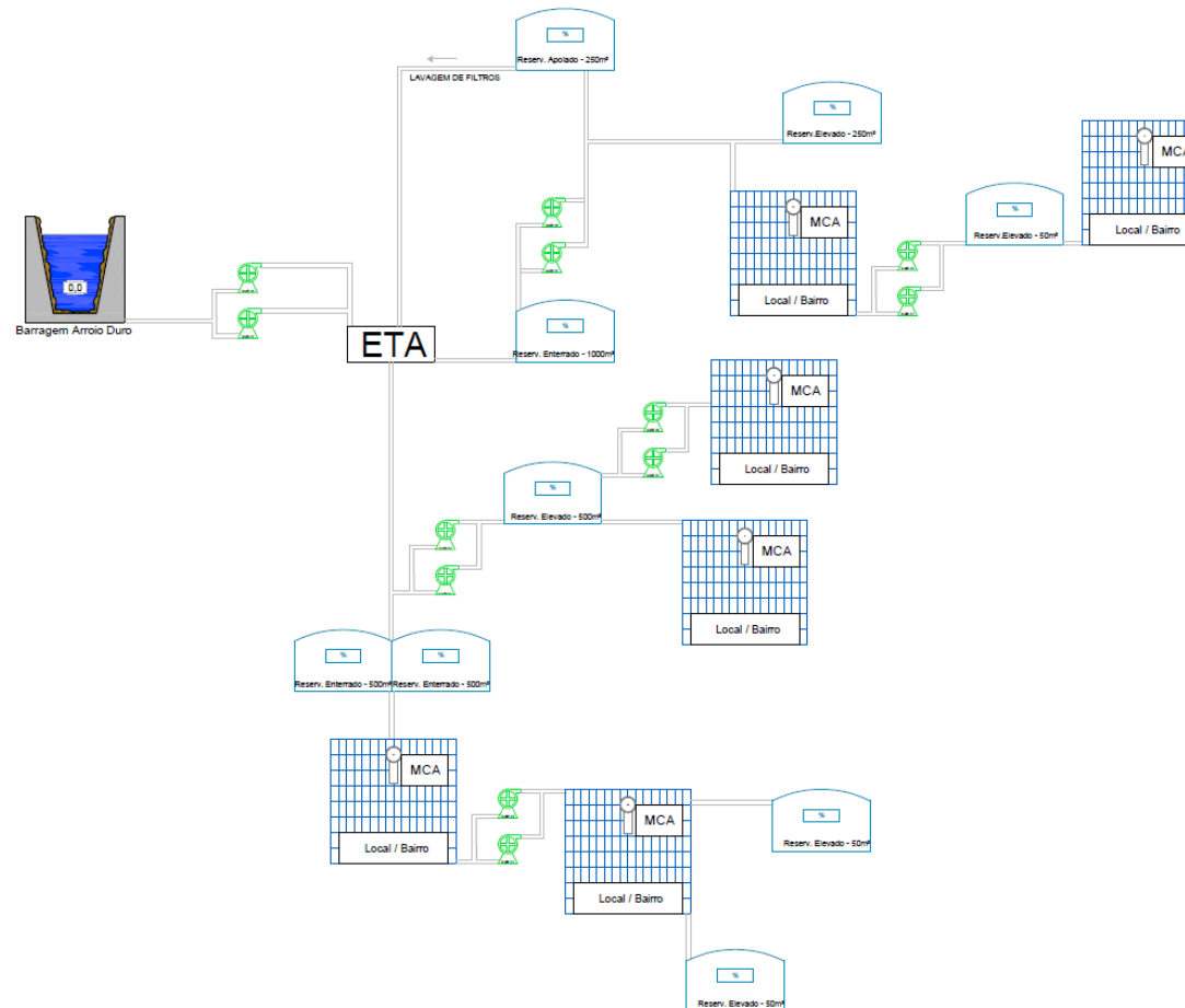
Figura 21 – Fluxograma do SAA.
