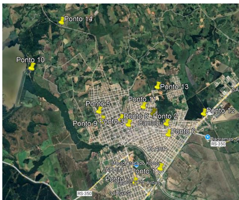
Figura 22 – Pontos vulneráveis do SAA (1).
