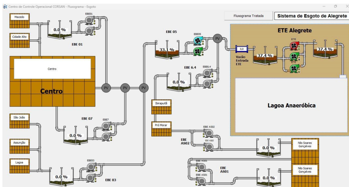
Figura 25 – Fluxograma simplificado do SES Alegrete atual.
