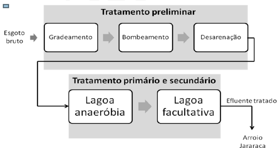
Figura 23 – Fluxograma simplificado do tratamento na ETE Ibirapuitã.
