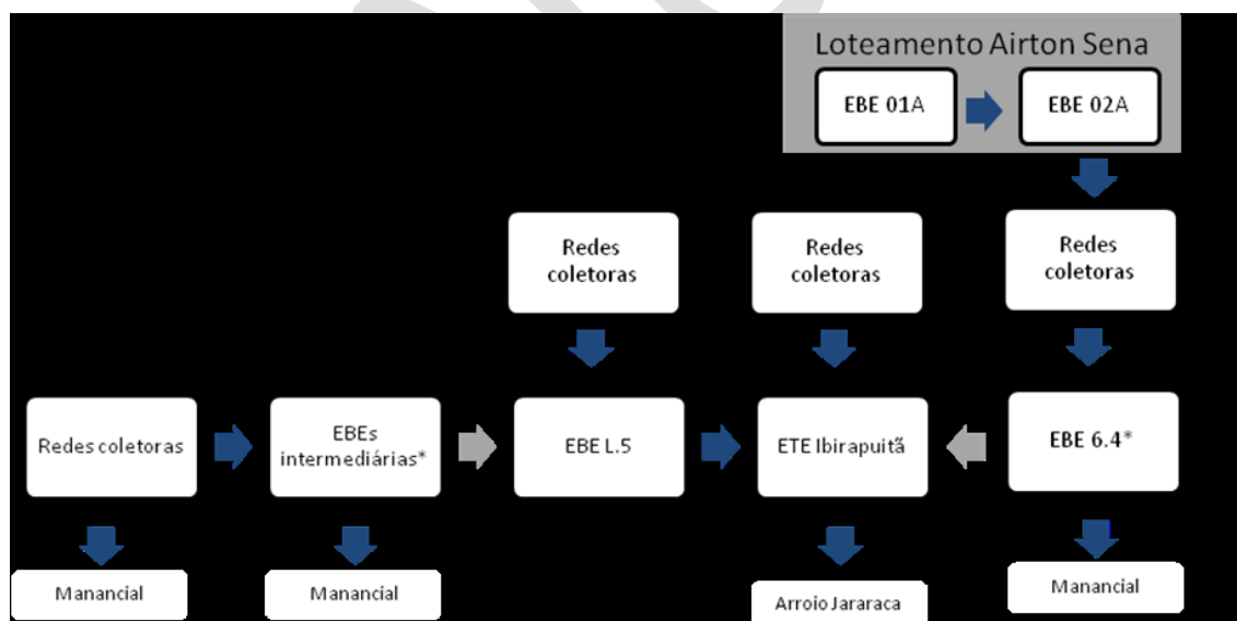
Figura 24 – Fluxograma simplificado do SES Alegrete.
