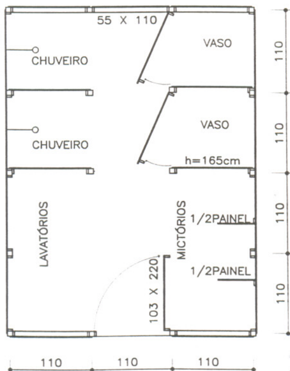
PLANTA BAIXA
