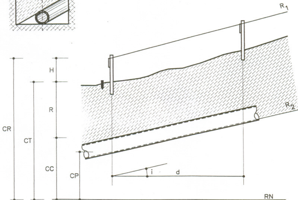
CORTE LONGITUDINAL
