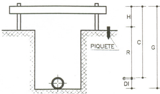
CORTE TRANSVERSAL
