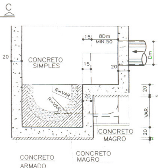
CORTE D-D
