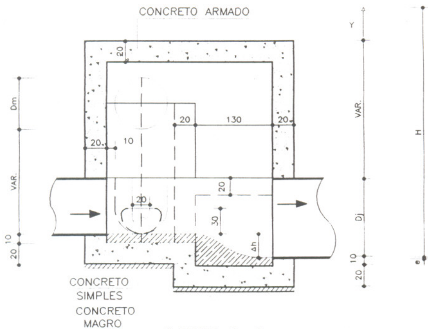
CORTE C-C
