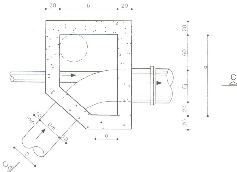
PLANTA BAIXA
