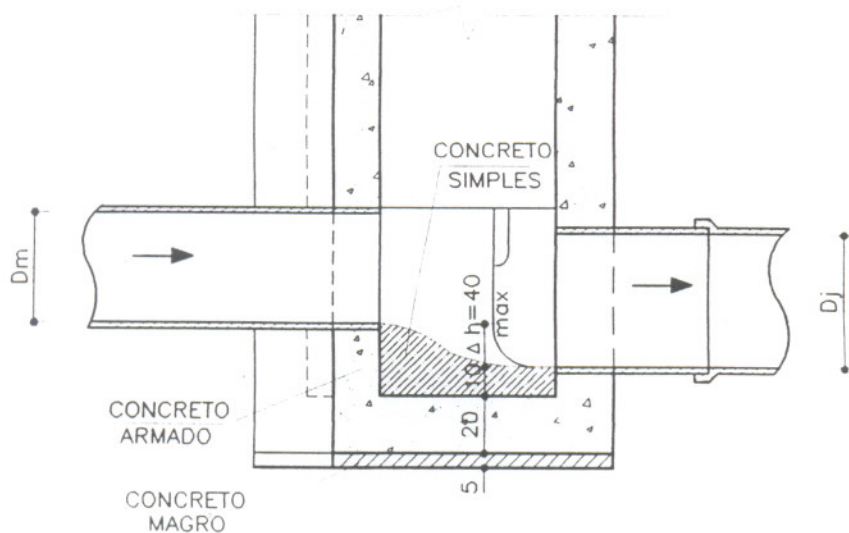
CORTE C-C
