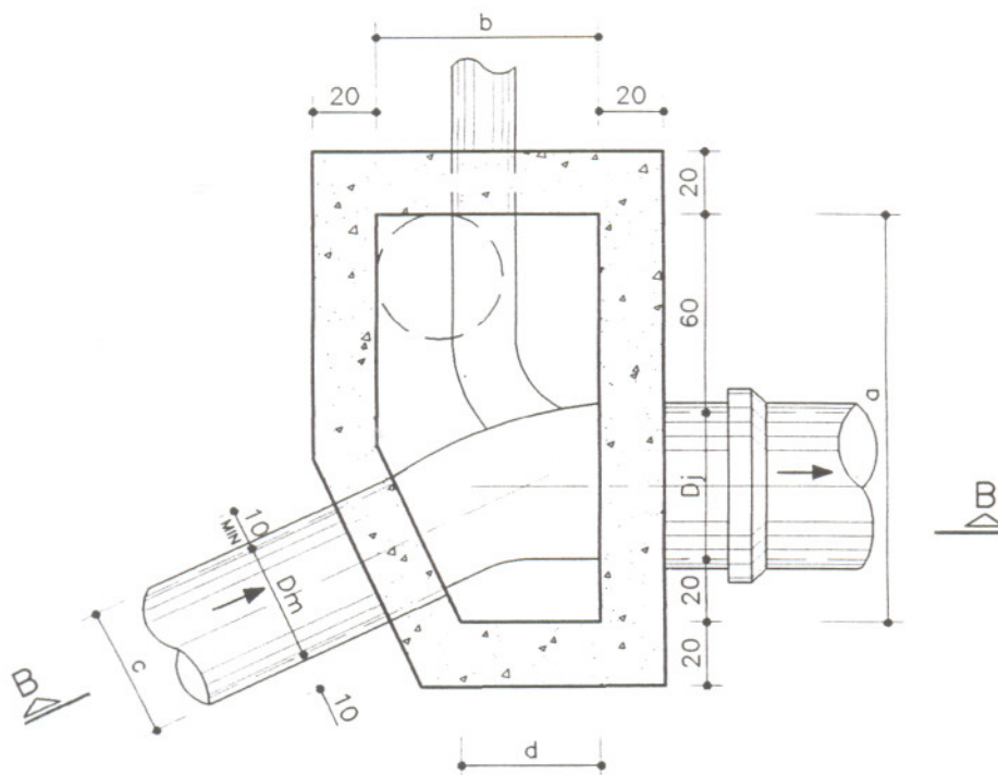
PLANTA BAIXA
