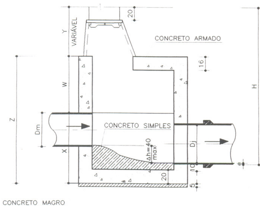
CORTE B-B
