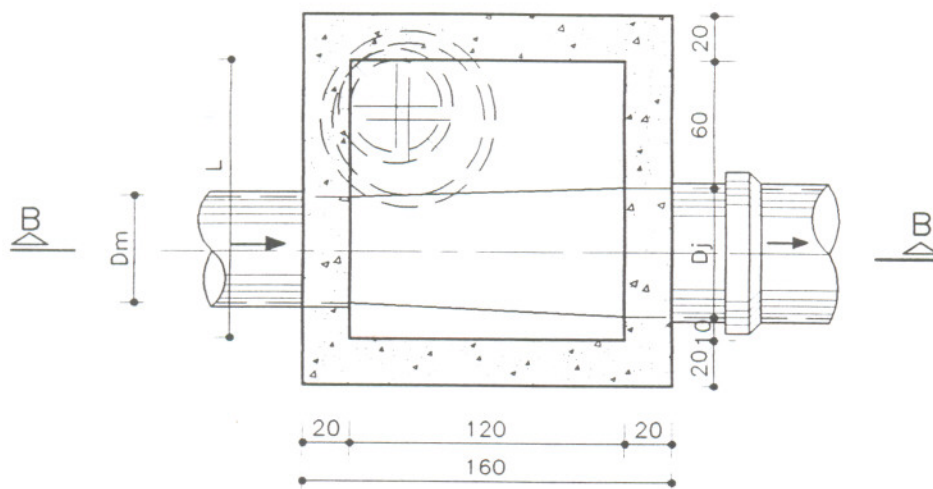
PLANTA-BAIXA
