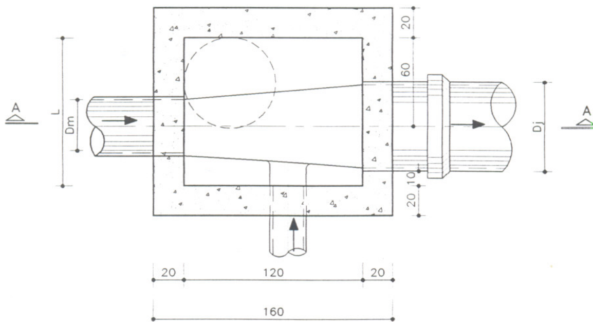
PLANTA-BAIXA
