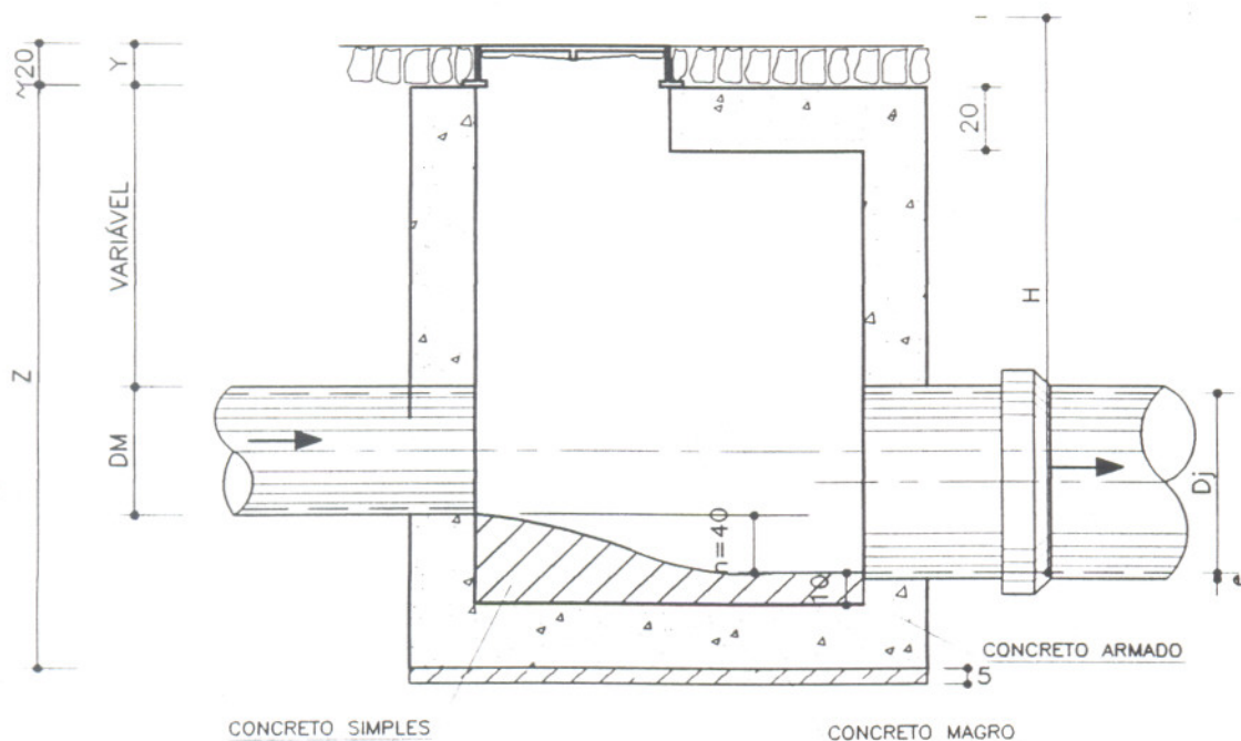
CORTE A-A
