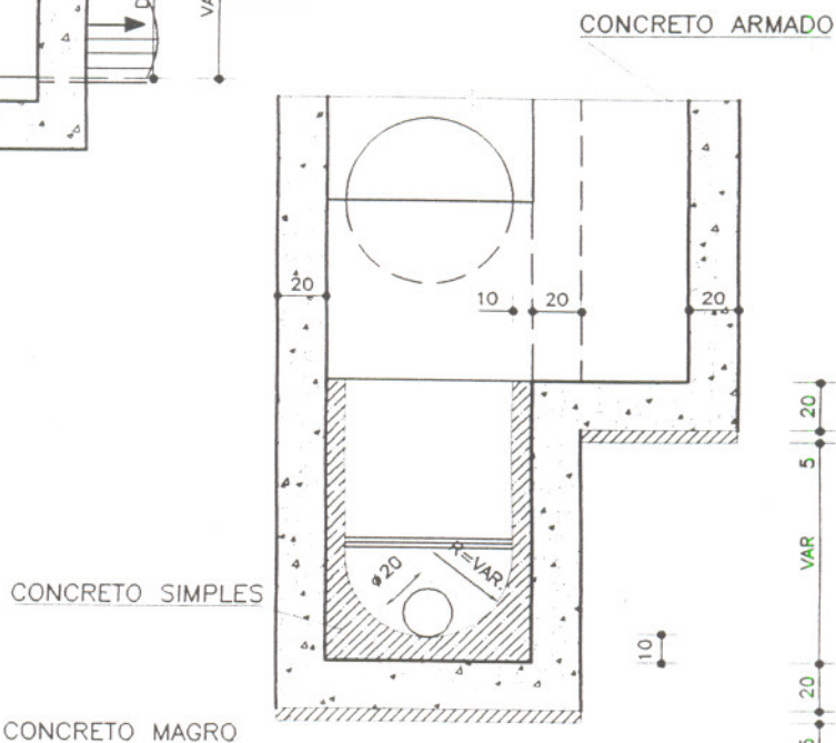
CORTE B-B
