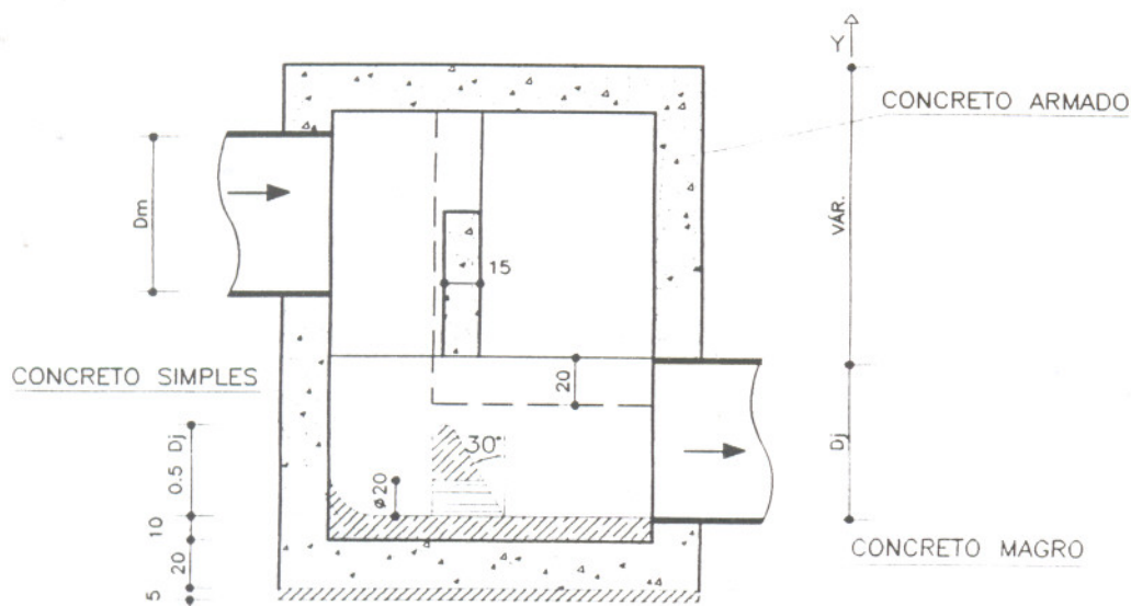
CORTE B-B
