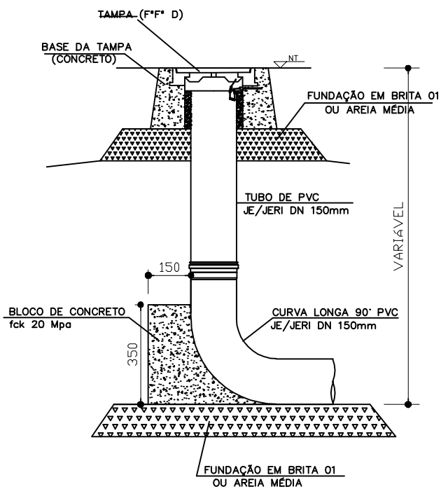
VISTA LATERAL
