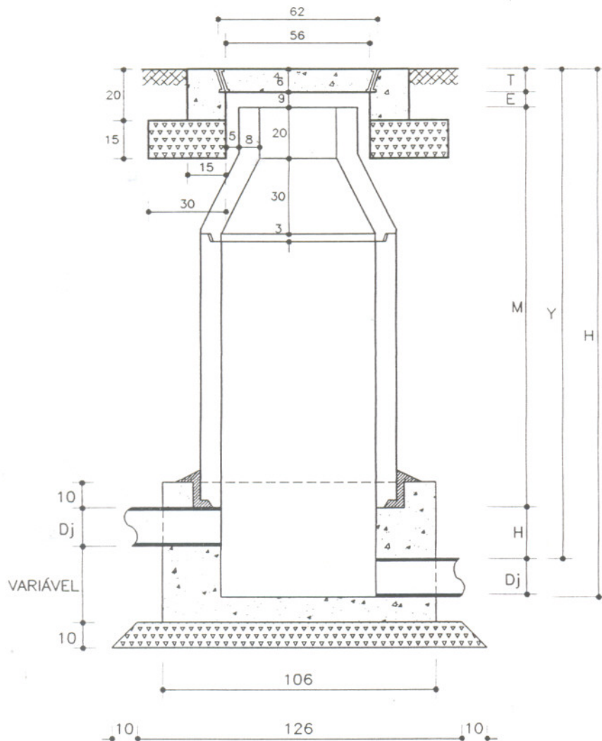
ESQUEMA GERAL
