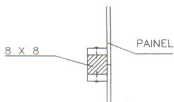
EM MONTANTE INTERMEDIÁRIO
