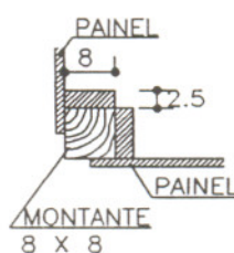
EM MONTANTE DE CANTO
