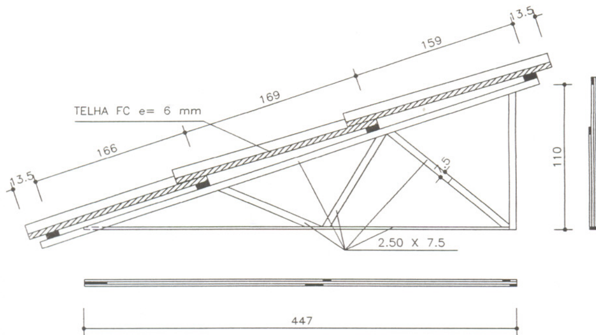
DETALHE DA FIXAÇÃO DOS PAINELIS
