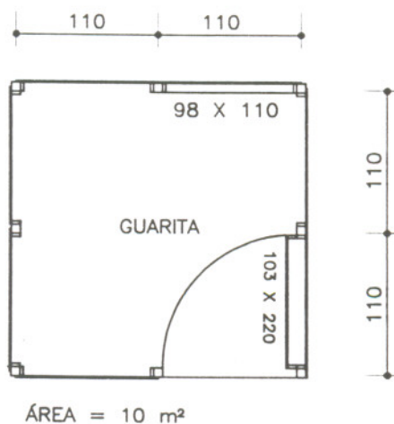
PLANTA BAIXA
