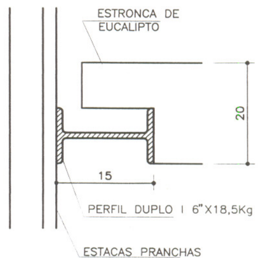
DETALHE
