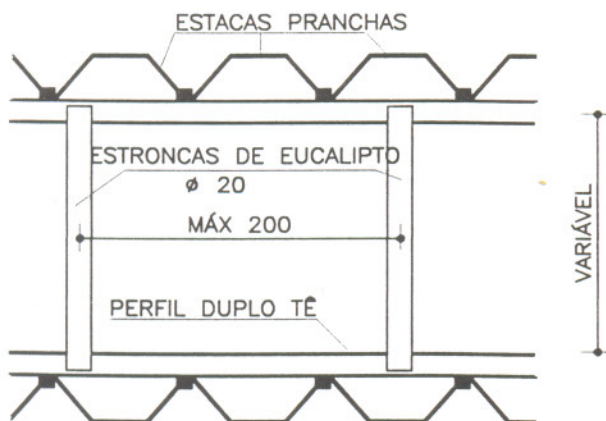
PLANTA- BAIXA
