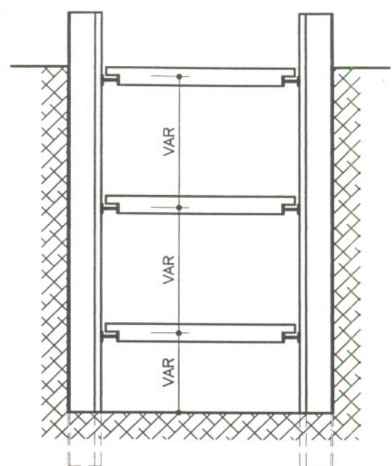
CORTE
