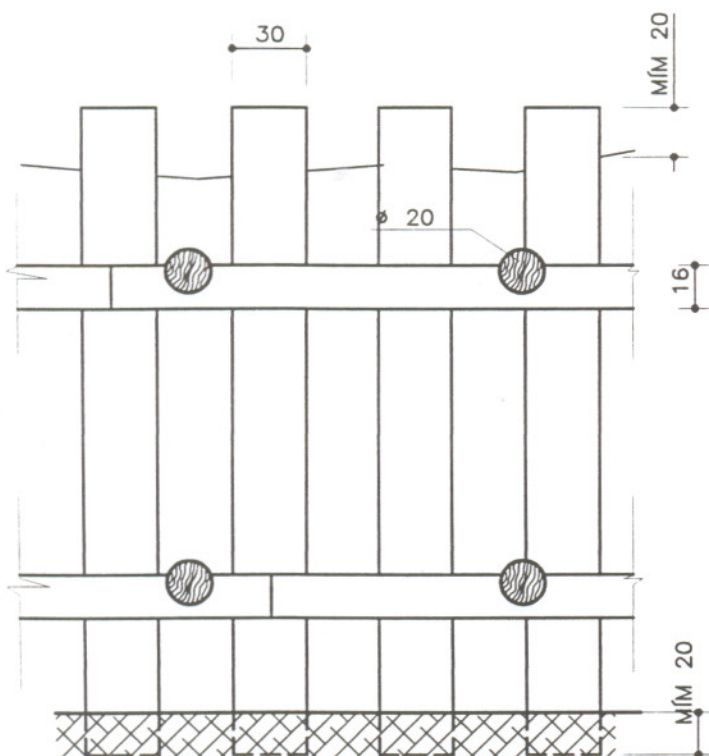
ELEVAÇÃO
