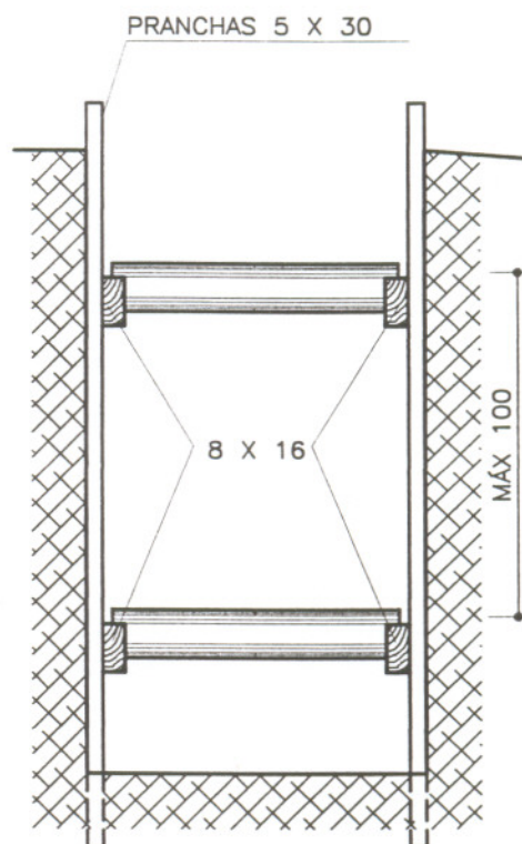
CORTE
