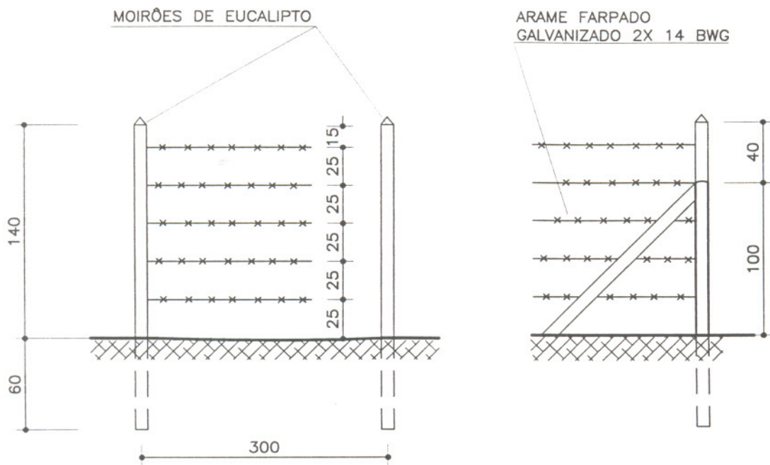
DETALHE DO REFORÇO DO CANTO DA CERCA
