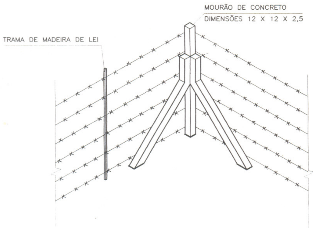
DETALHE DE MUDANÇA DE DIREÇÃO
