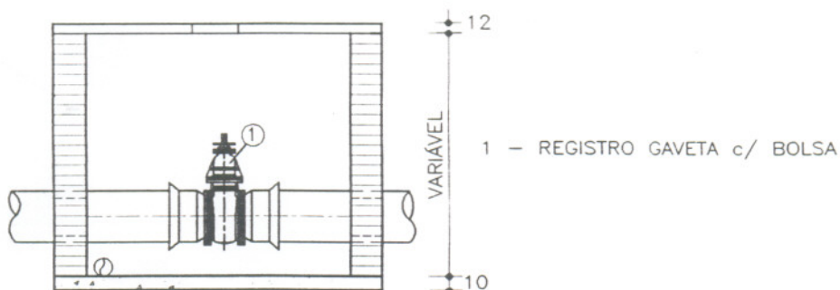
ELEVAÇÃO
