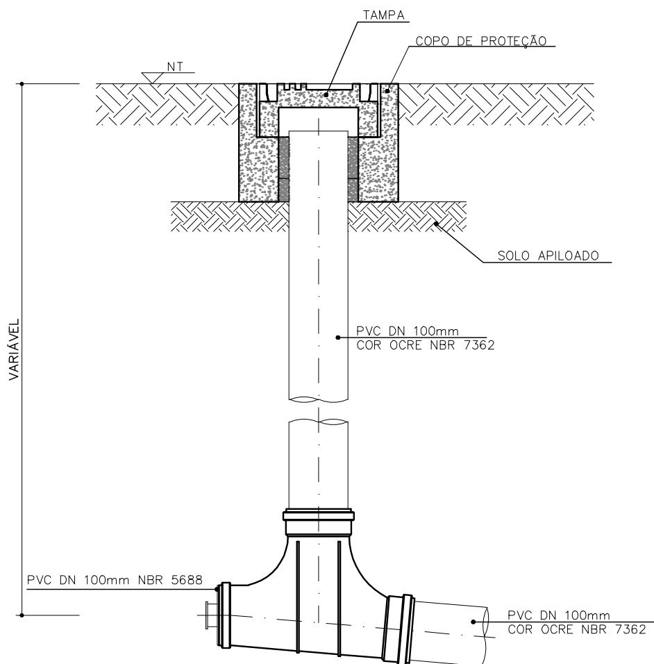
DETALHE DA CAIXA DE CALÇADA COM TIL JE DE LIGAÇÃO PREDIAL DN 100 mm
