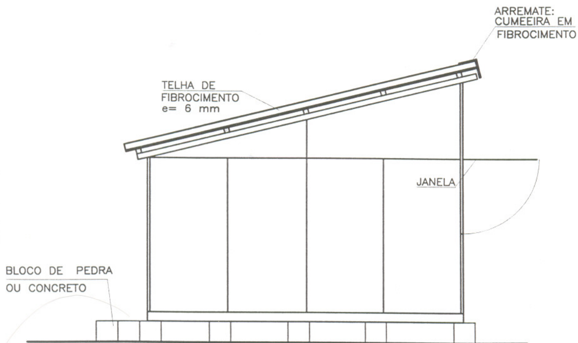
VISTA LATERAL
