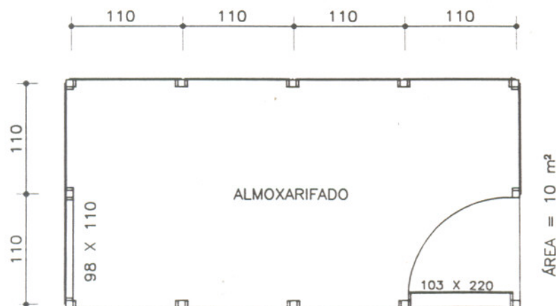
PLANTA BAIXA
